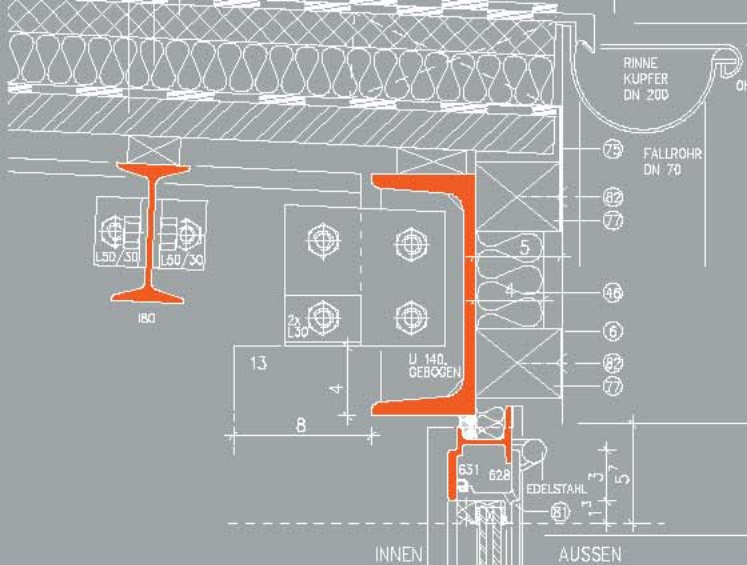
Detail: Wintergarten, ehem. Bundesschule des ADGB in Bernau, 2004 (Zeichnung: Brenne GmbH)
